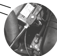
Unterbrecherkontakt einstellen /Adjusting Breaker Point Gap 914-6
