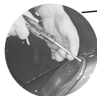
Fernscheinwerfer Glühbirne wechseln/ Replacing Driving Light Bulb
